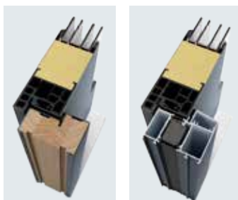
Ościeżnica met/drew
