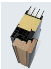
Ościeżnica met/drew
